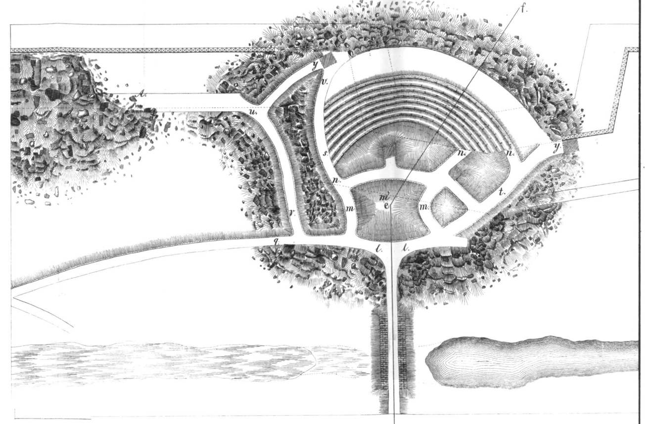
Планъ коронованія воронки II бастіона. № 4.
